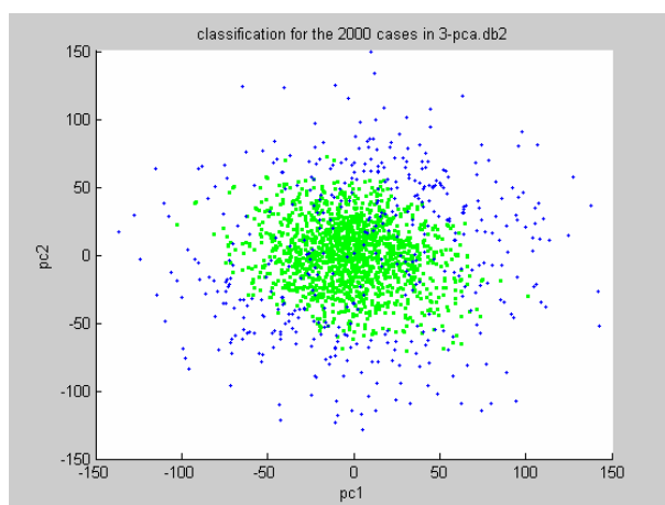
圖十七 PCA 圖【以前幾個主成分分類後，用第一及第二主成分所繪製的資料分布圖】
