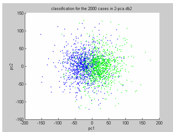
圖十六 PCA 圖【圖十五的兩千筆動作電位經 PCA 轉換後，以第一及第二主成分所繪製的資料分布圖】
